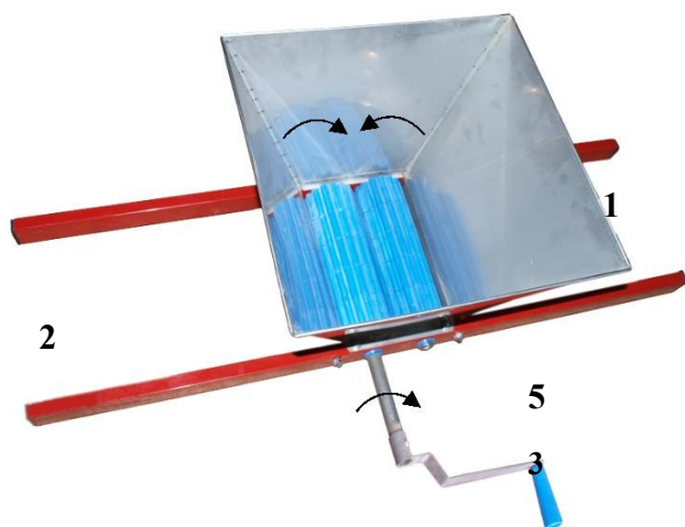
obr. 1 - drcení hroznů
